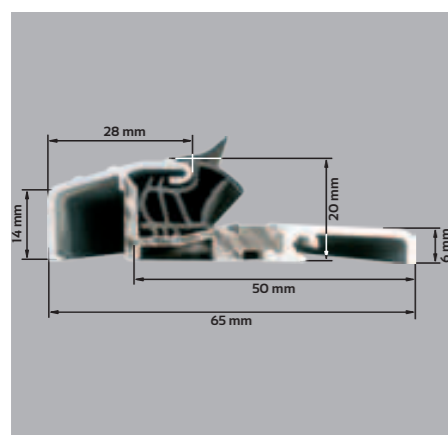
PRÓG ALUMINIOWY Z WŁĄDKĄ TERMICZNĄ
