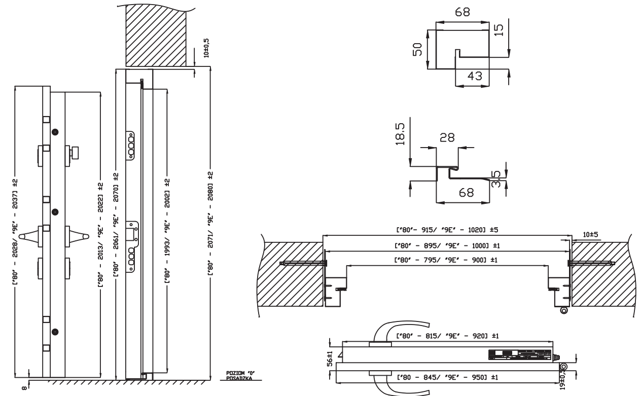
WYMIARY I PRZEKROJE DRZWI I OŚCIEŻNICY METALOWEJ
