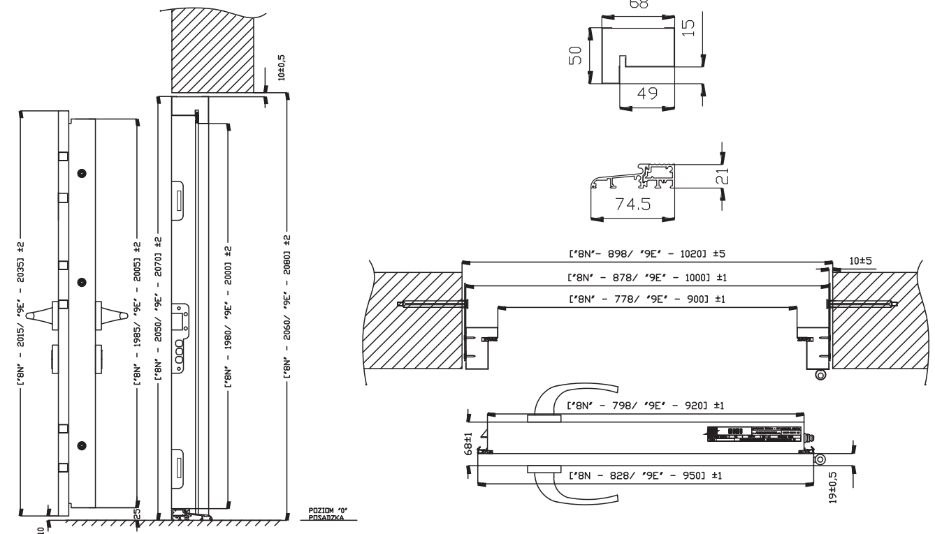
WYMIARY I PRZEKROJE DRZWI I OŚCIEŻNICY METALOWEJ
