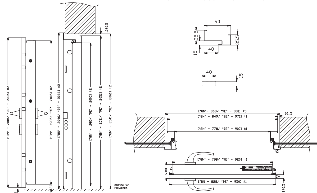
WYMIARY I PRZEKROJE DRZWI I OŚCIEŻNICY METALOWEJ
