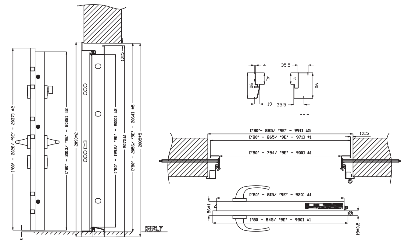
WYMIARY I PRZEKROJE DRZWI I OŚCIEŻNICY METALOWEJ
