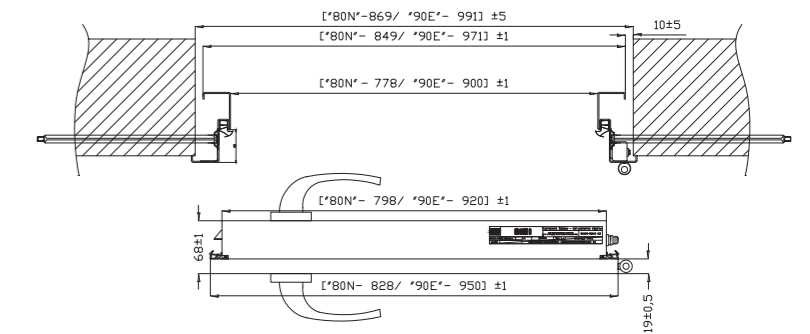
WYMIARY I PRZEKROJE DRZWI I OŚCIEŻNICY METALOWEJ
