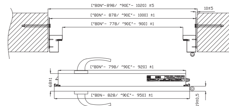
WYMIARY I PRZEKROJE DRZWI I OŚCIEŻNICY ENERGO
