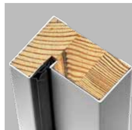
PRZEKRÓJ OŚCIEŻNICY
